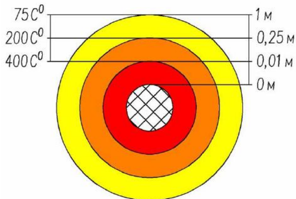
Температурные зоны АГС 11/5÷6
